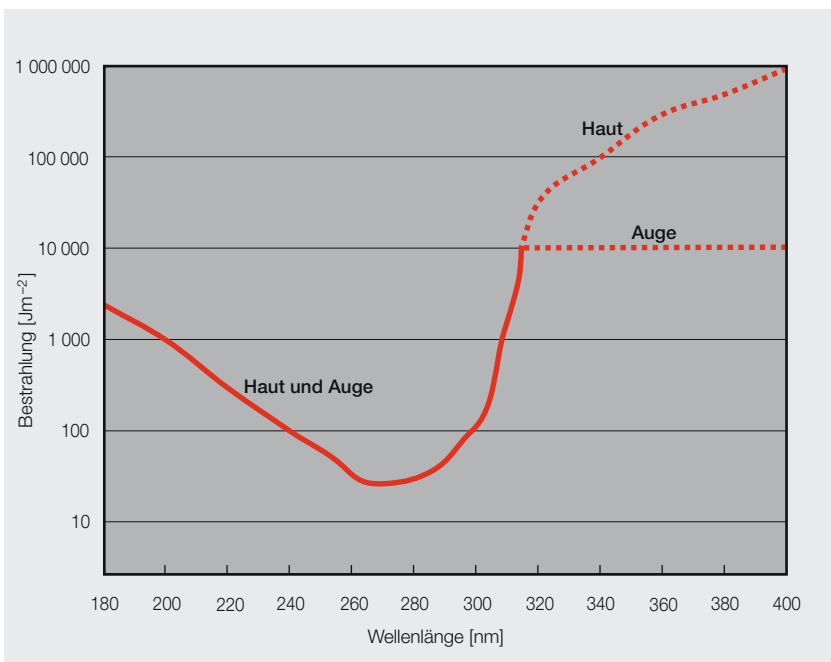
Figur 1 UV-Strahlungs-Grenzwerte innerhalb von 8 Stunden (Arbeitstag). Graphische Darstellung der Bestrahlungsgrenzwerte aus Tabelle 2 (Seite 142).
